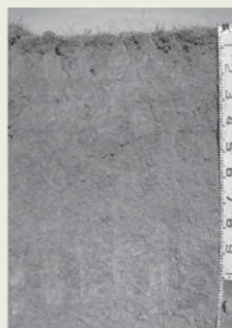
Black Dermosol
